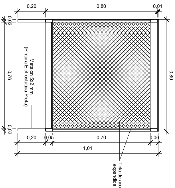
2 CORTE A 1 : 10
